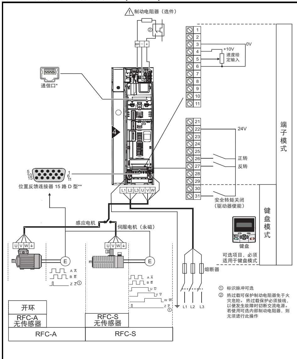
图 6-1 电机以任何模式运行的最小连接 (所示 4 型)
