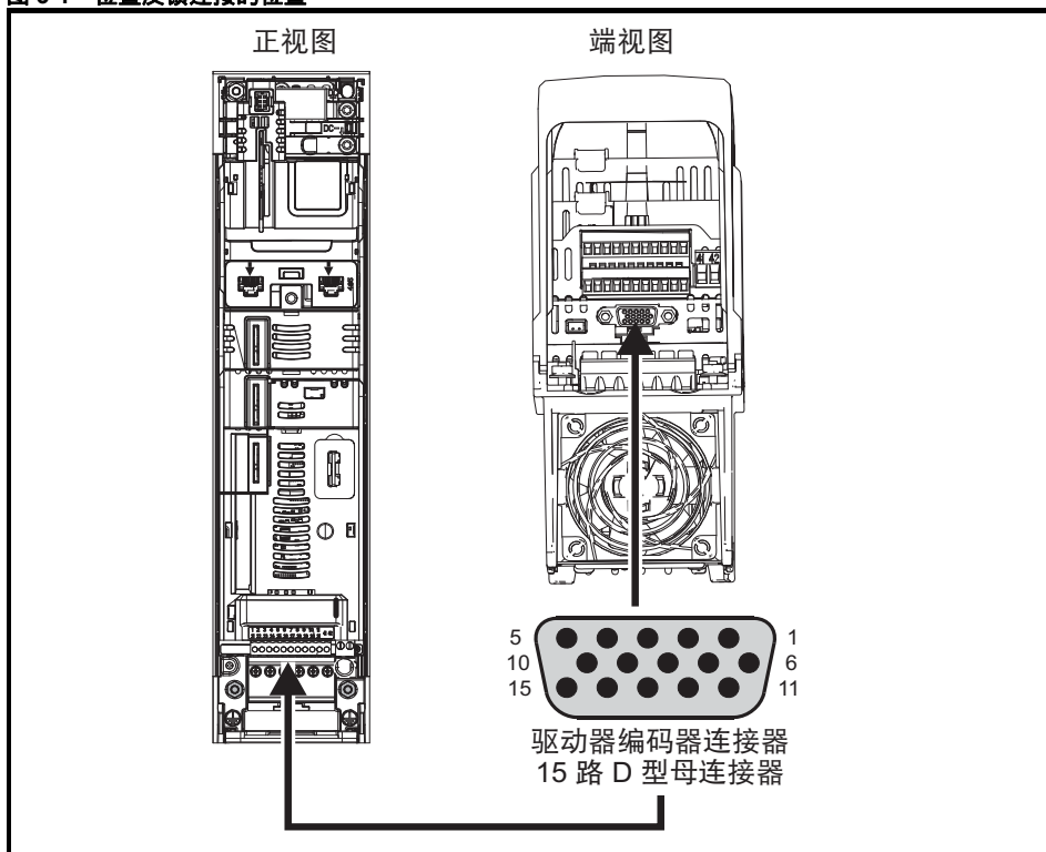
图 3-1 位置反馈连接的位置
