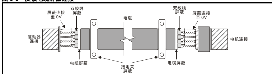
图 3-5 反馈电缆屏蔽连接
