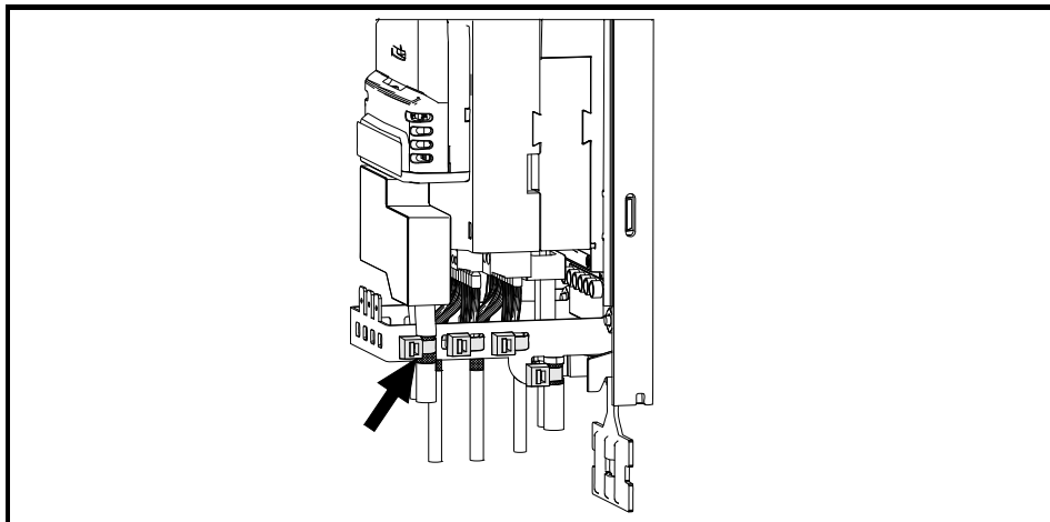
图 3-4 使用接地支架将信号电缆屏蔽接地
