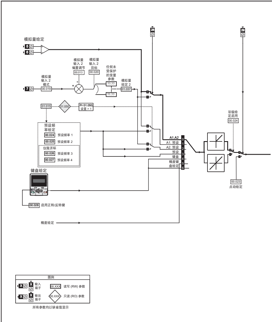
图 5-1 菜单 0 逻辑图
