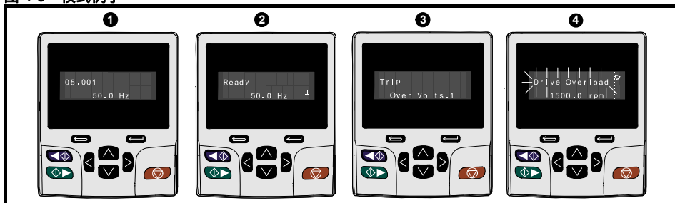
图 4-3 模式例子
