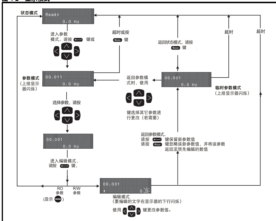
图 4-2 显示模式
