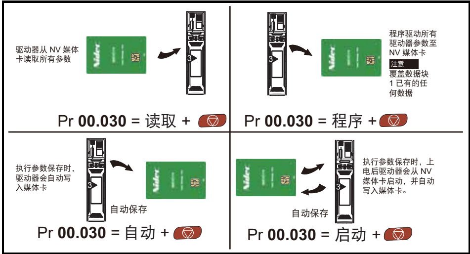
图 4-6 基本 NV 媒体卡操作
